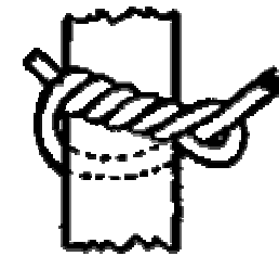
Nudo de Leñador. Para asegurar el cabo de una cuerda a un mástil o tubería
