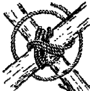
Amarre Diagonal. Comiéndose con el nudo de leñador alrededor de los dos postes. Déense vueltas alrededor para atortolar (apretar). Termínese con el ballestrinque.
