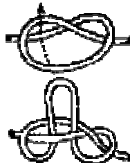
Nudo de Arnés de hombre. Hace una gaza para arrastre o soportes intermedios en sistemas de guía (tirolesas y rieles)
