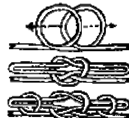
Nudo de Silla de Bombero. Tiene dos gazas para bajar personas.
